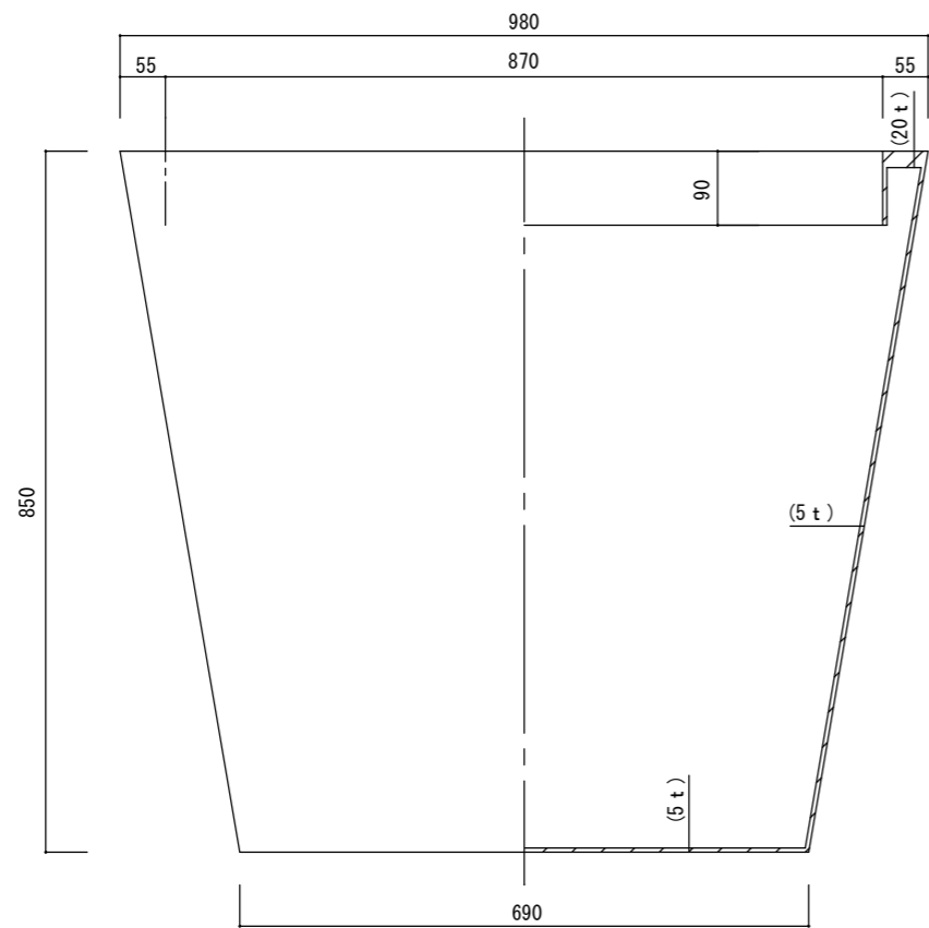
立・断面図
