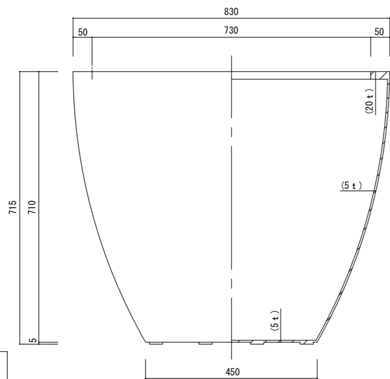
立・断面図
