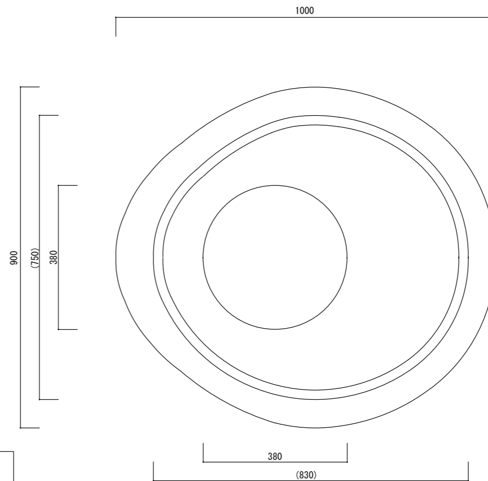
底面図
