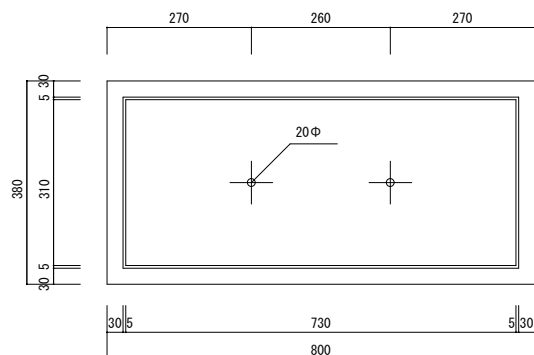
底面図
