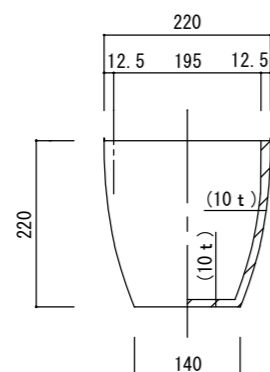
立・断面図
