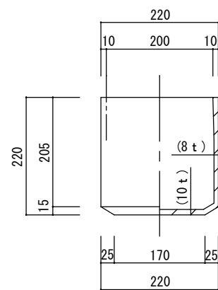
立・断面図
